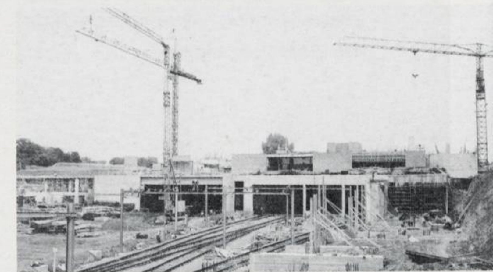
Bouw van de spoorlijn naar Louvain-La-Neuve, in die periode een vernieuwende vorm van stedenbouwkunde.
